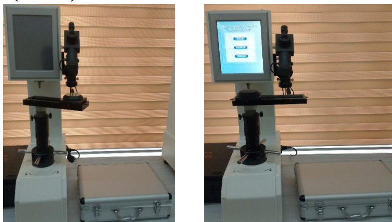
1-rasm. THBRV-187.5DX qattqlikni o'lchash qurilmasining umumiy ko'rinishi
