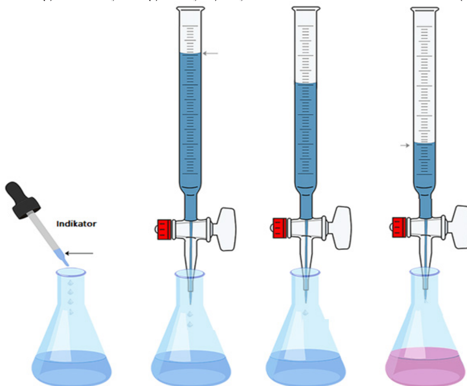
1-rasm. Titrlash yordamida aniq konsentratsiyali ishqor bilan noaniq konsentratsiyali kislotani miqdorini aniqlash
